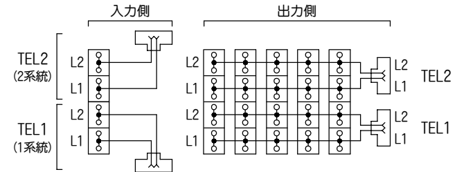
回路図
